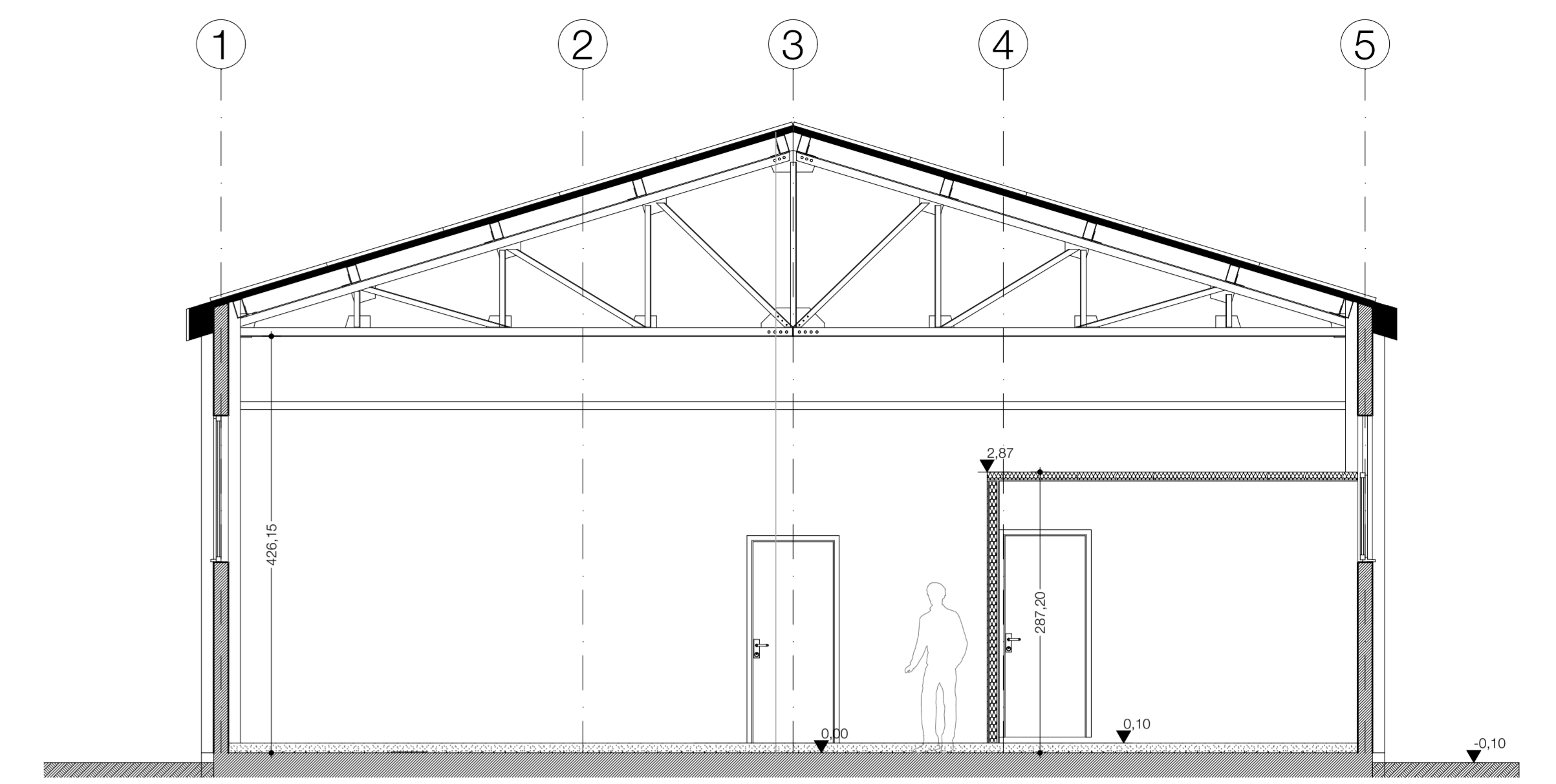
SEZIONE S1 STATO DI PROGETTO
